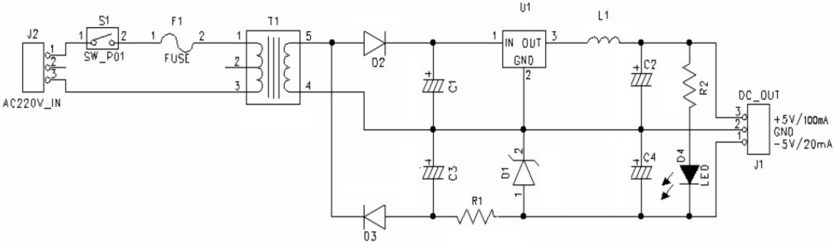
(전원공급장치 회로도)
