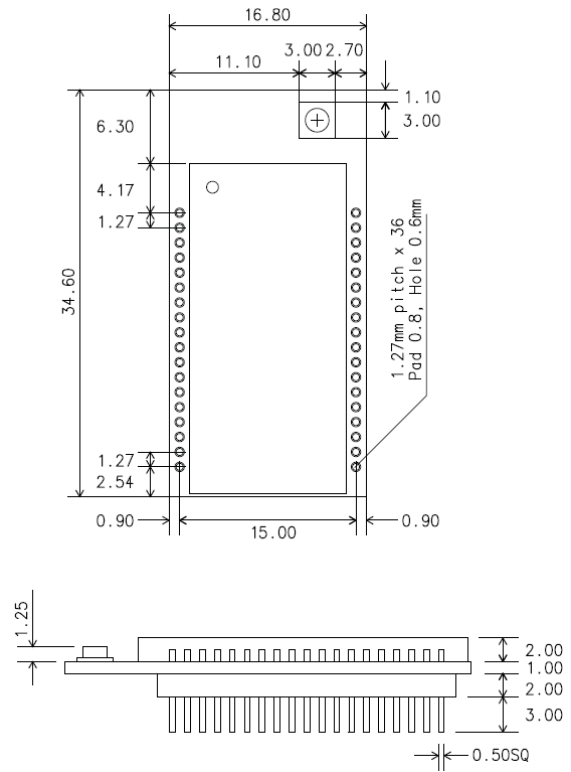
그림 1-4 BCD110DU 치수
