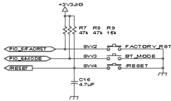
그림 5-5 스위치 인터페이스
