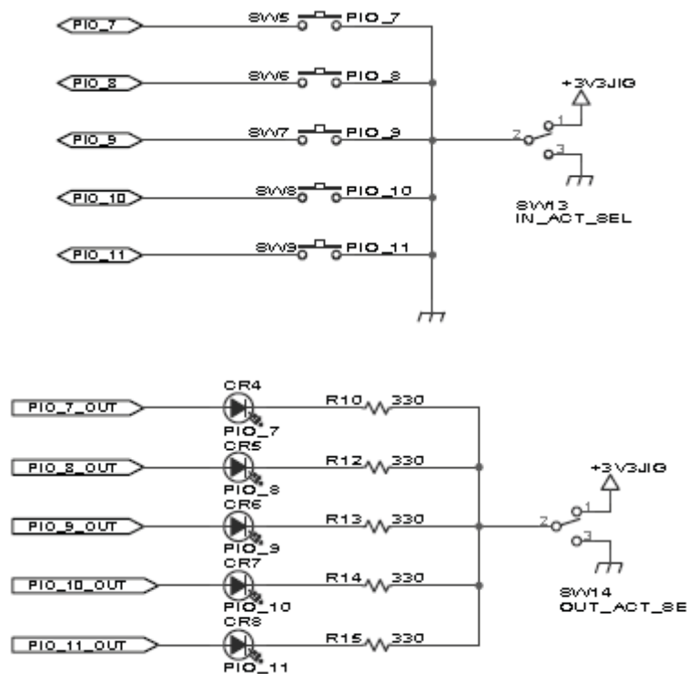
그림 5-6 GPIO 인터페이스
