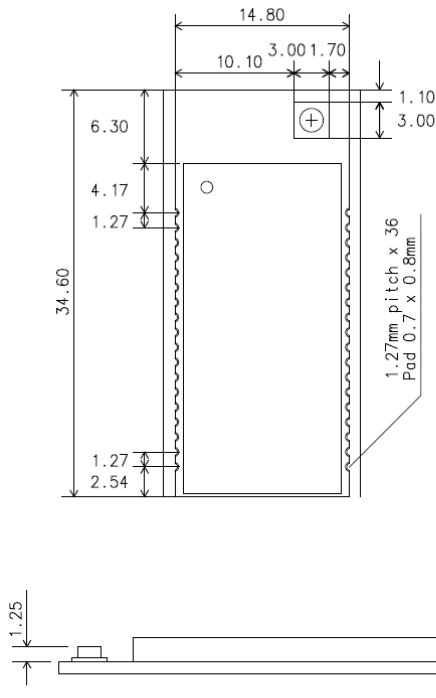
그림 1-3 BCD110SU 치수
