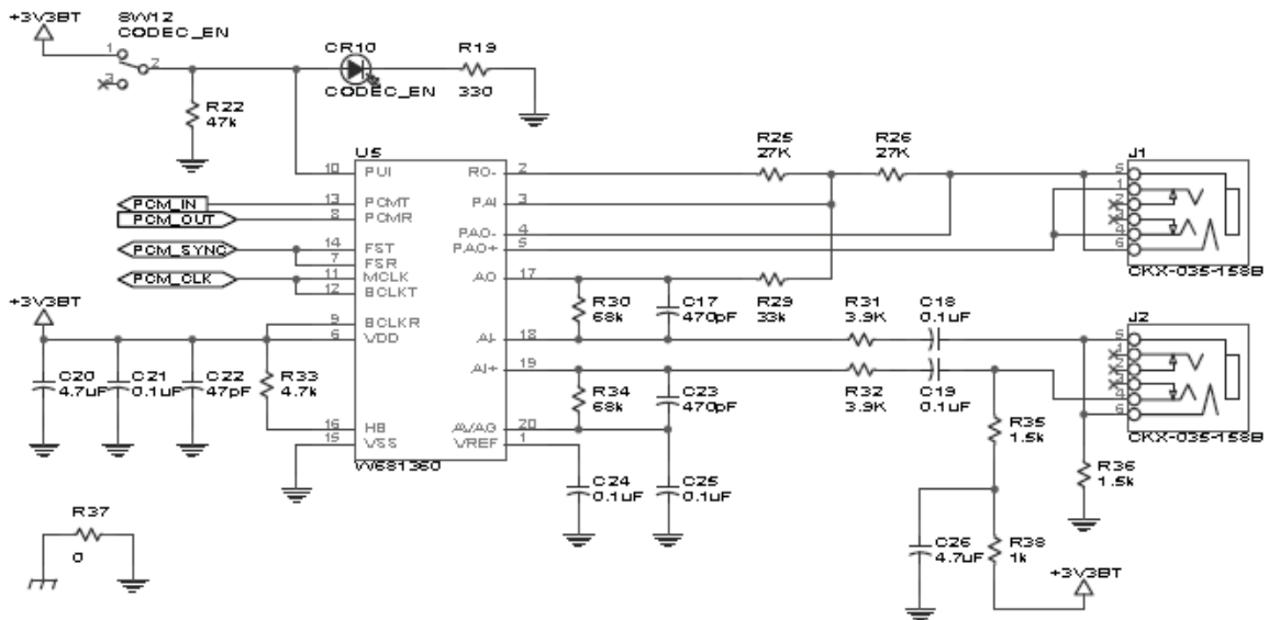
그림 5-9 PCM 인터페이스
