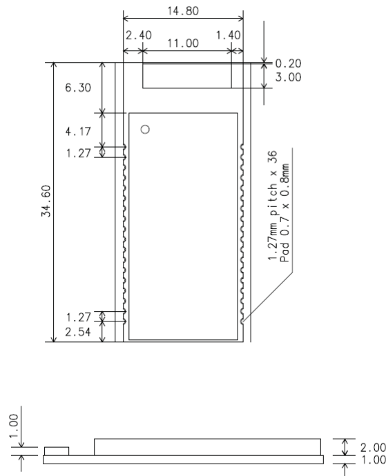
그림 1-3 BCD110SU 치수
