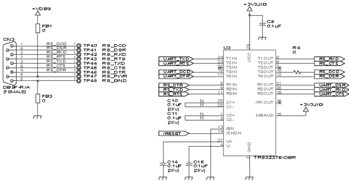
그림 5-3 RS232 시리얼 인터페이스
