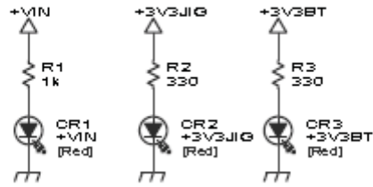
그림 5-8 LED 인터페이스
