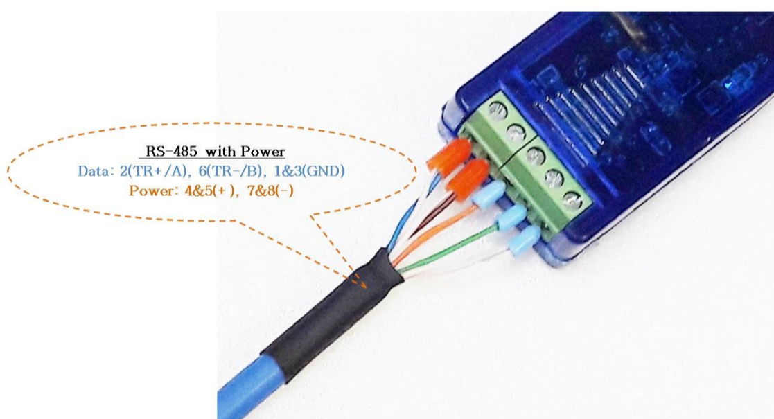
터미널 블럭형 RS-485 장비 결선
