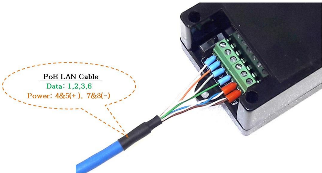
터미널 블럭형 PD(Powered Device) 결선
