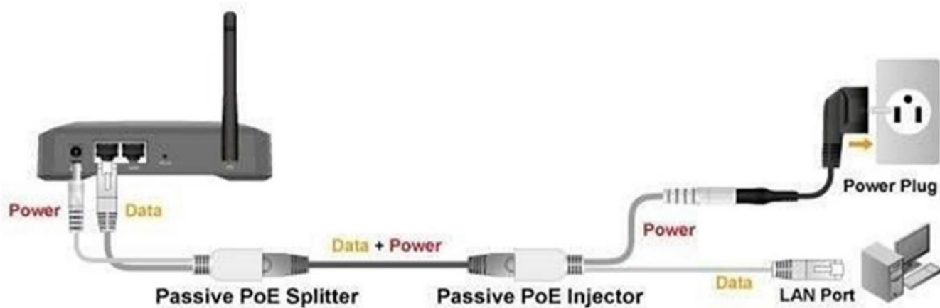
Passive PoE Adapter 사용
