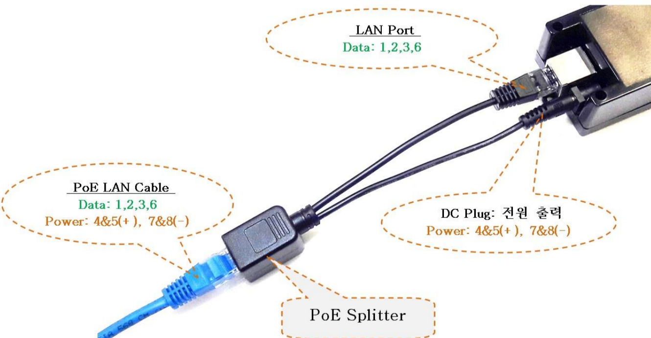
RJ-45 & DC Jack 사용 PD(Powered Device) 결선
