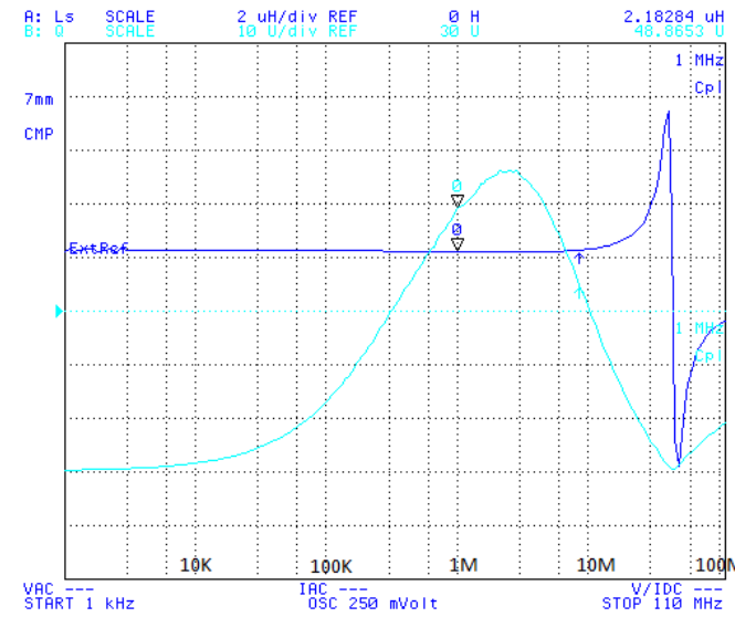
PIC252012-2R2
