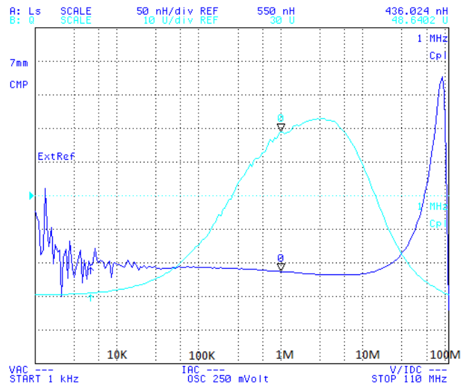
PIC252012-1R0
