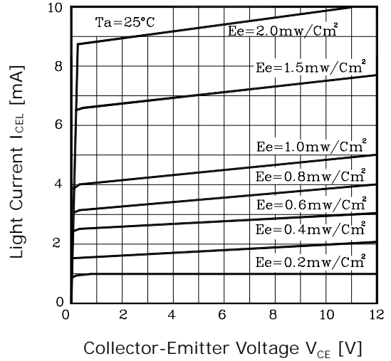
Fig. 2 I_{CEL} - V_{CE}
