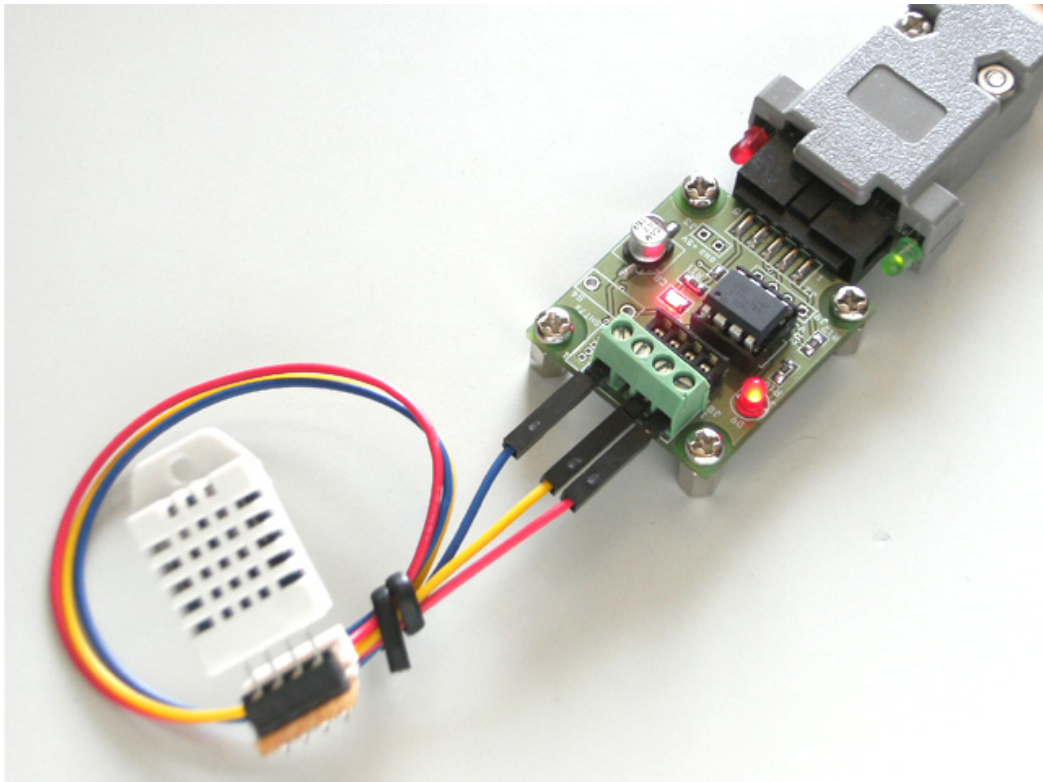
(온습도센서 CM2302 + USB232-RHT 모듈 + USB232-TTL )
