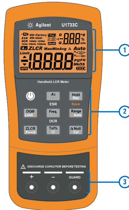
그림 1-7 전면판
