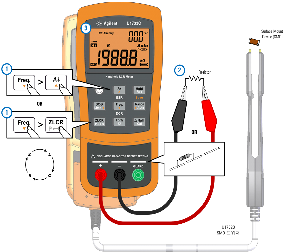
그림 2-7 저항 측정
