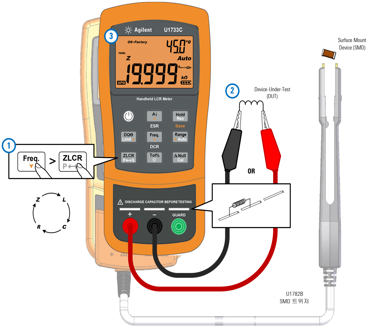
그림 2-9 임피던스 측정
