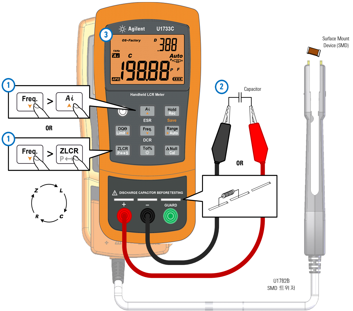
그림 2-5 캐패시턴스 측정
