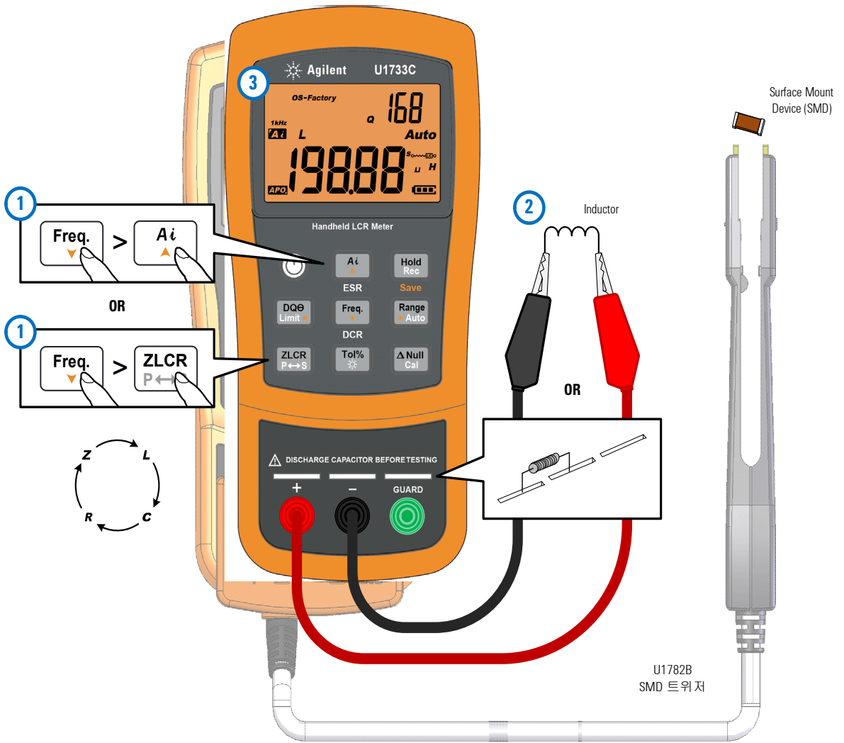
그림 2-3 인덕턴스 측정
