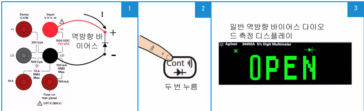
그림 1-16 역방향 바이어스 다이오드 단자 연결 및 디스플레이
