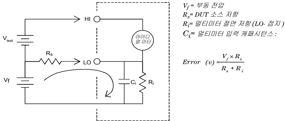
그림 3-1 CMR( 일반 모드 제거 )
