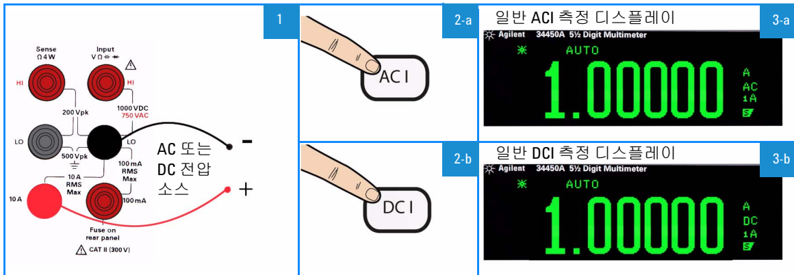
그림 1-10 ACIrms 또는 DCI(A) 단자 연결 및 디스플레이
