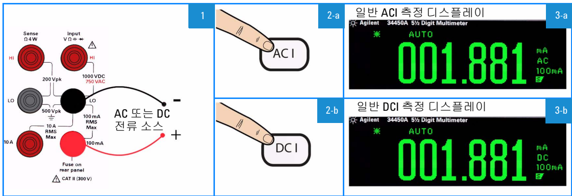
그림 1-9 ACIrms 또는 DCI(mA) 단자 연결 및 디스플레이
