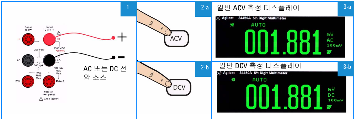
그림 1-6 ACV rms 및 DCV 단자 연결 및 디스플레이
