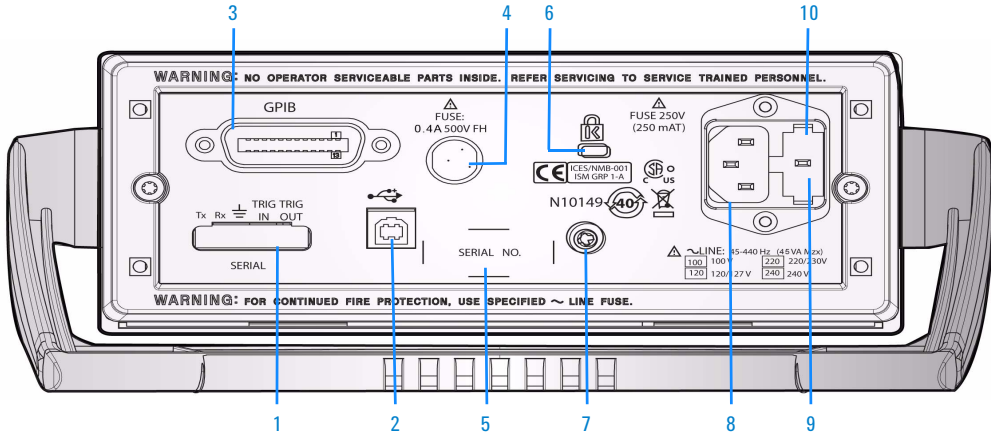
그림 1-5 후면 패널 개요
