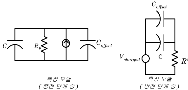
그림 3-6 캐패시터에 전류 적용
