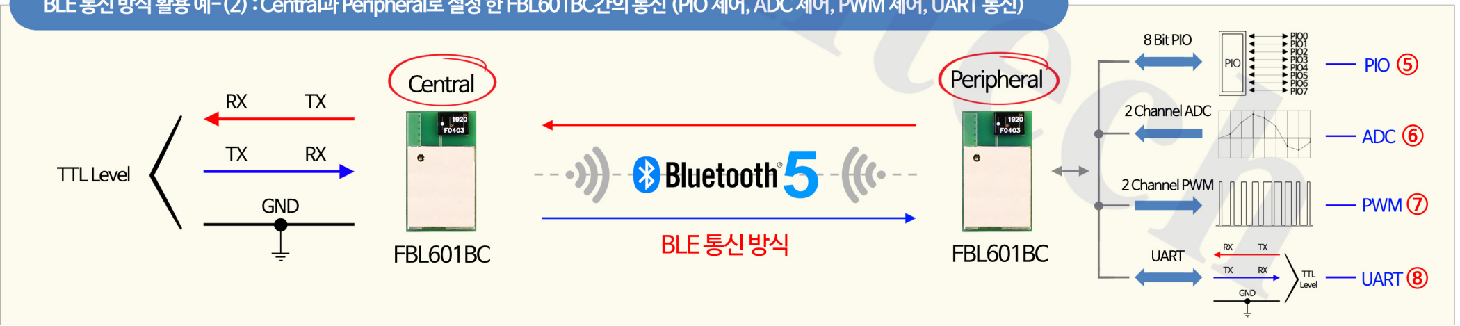
BLE 통신 방식 활용 예-(2) : Central과 Peripheral로 설정 한 FBL601BC간의 통신 (PIO 제어, ADC 제어, PWM 제어, UART 통신)
