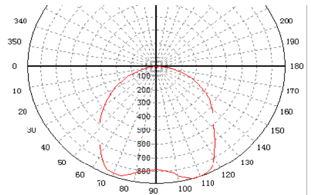
角度-光强 极坐标分布图
