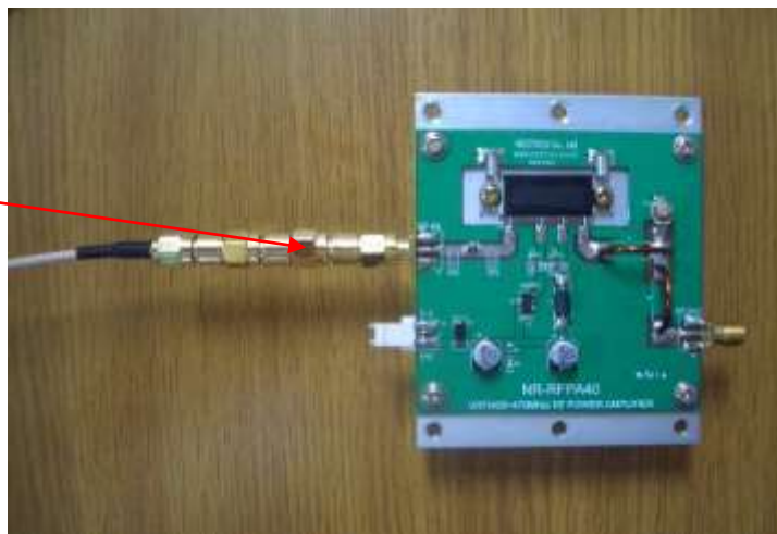
(여러 개의 감쇄기를 직렬로 연결하여 감쇄기의 용량을 늘린 모양)
